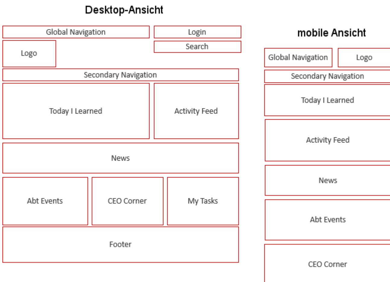
Abbildung: Responsive-Design - Desktop- Ansicht vs. mobile Ansicht[3]
