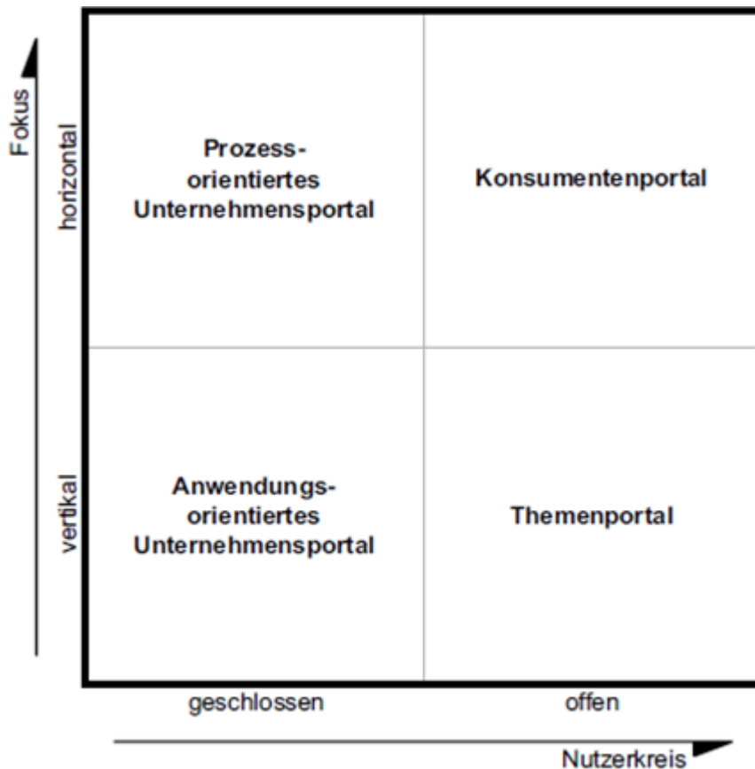
Abbildung: Kategorisierungsmatrix[2]
